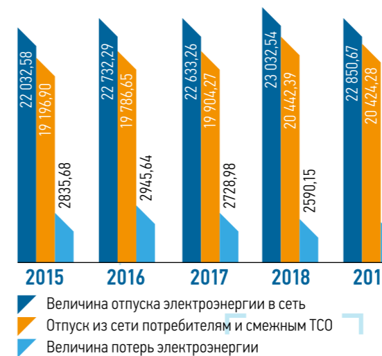
ОТПУСК ЭЛЕКТРОЭНЕРГИИ В СЕТЬ И ИЗ СЕТИ ПАО «КУБАНЬ-ЭНЕРГО» И ПОТЕРИ ПРИ ПЕРЕДАЧЕ ЭЛЕКТРОЭНЕРГИИ, МЛН КВТ·Ч:
