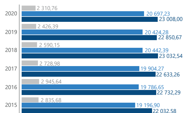
Отпуск электроэнергии в сеть из сети ПАО «Россети Кубань» и потери при передаче электроэнергии (млн кВт • ч)
